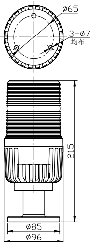
法兰盘安装
