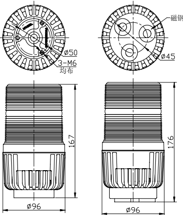
常规安装
