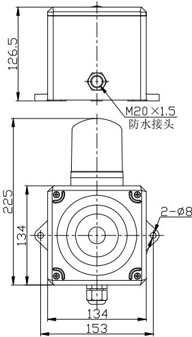
安装尺寸图 (单位: mm)
