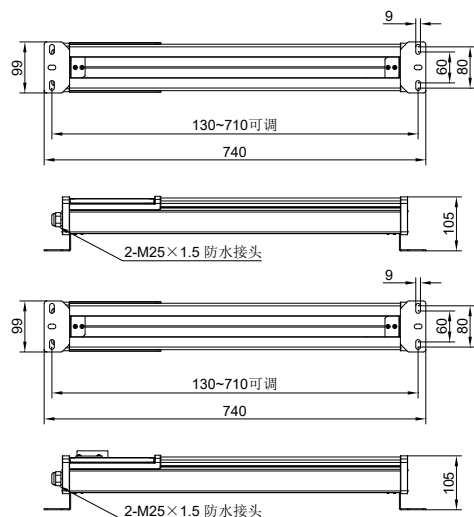
安装尺寸图 (单位: mm)
