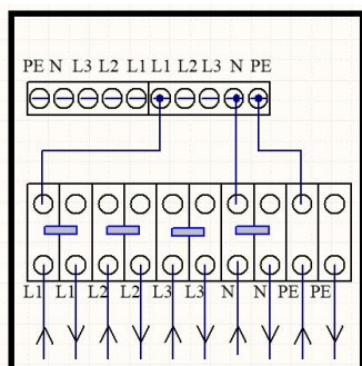
接线端子示意图
