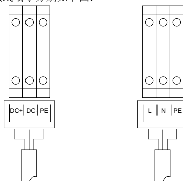
FR104 控制器接线示意图
