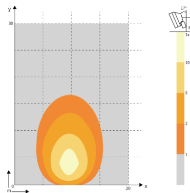
14W 1600lm
